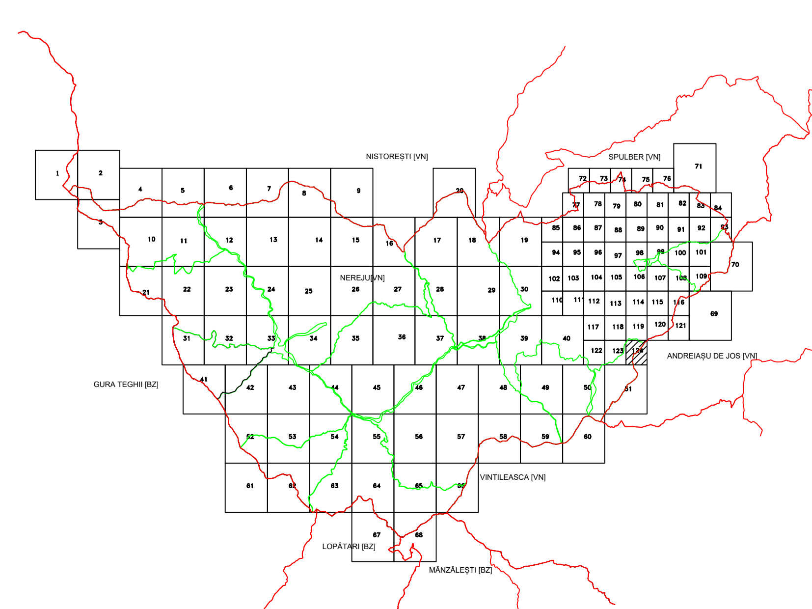
Schema planșelor
