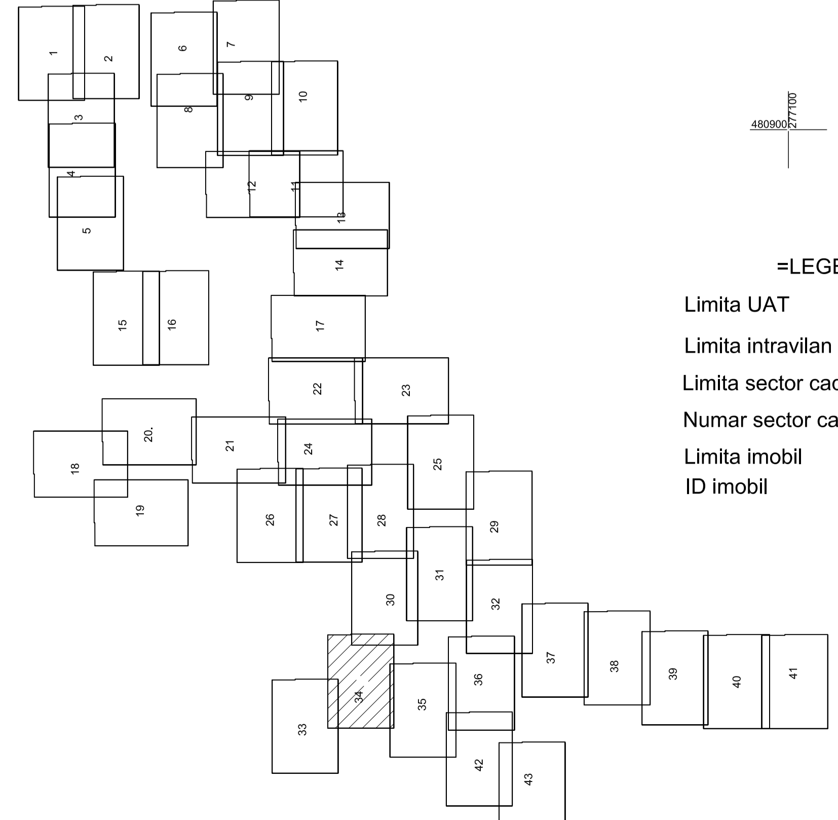
schita de racordare a planselor
