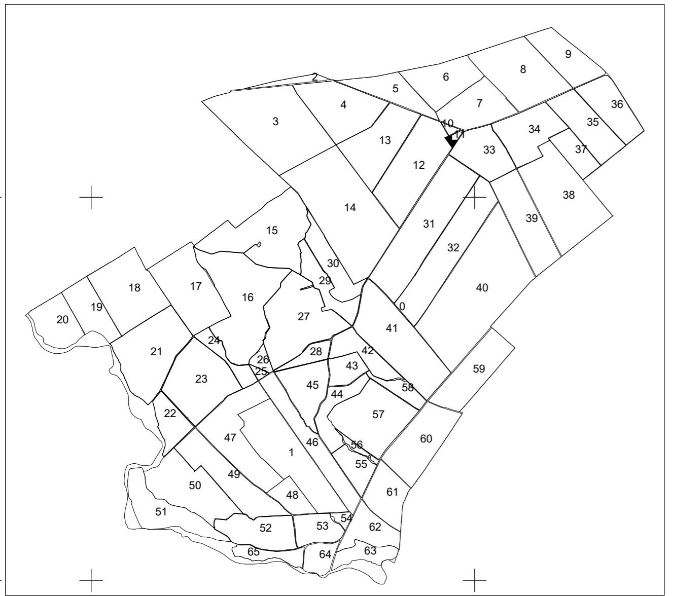
SCHEMA DE DISPUNERE A SECTOARELOR CADASTRALE
