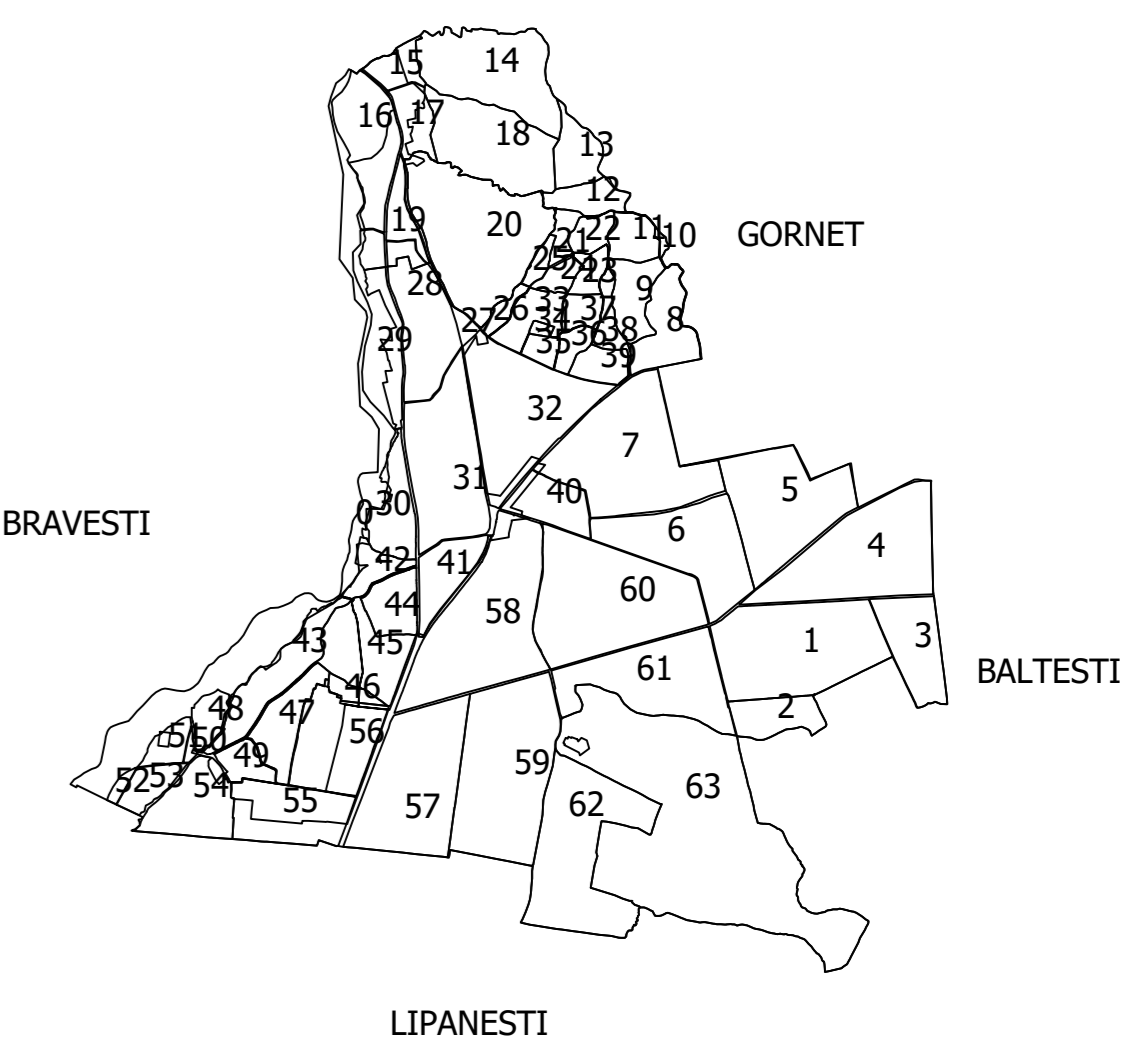
GURA VIITIOAREI Schita cu dispunerea sectorului
