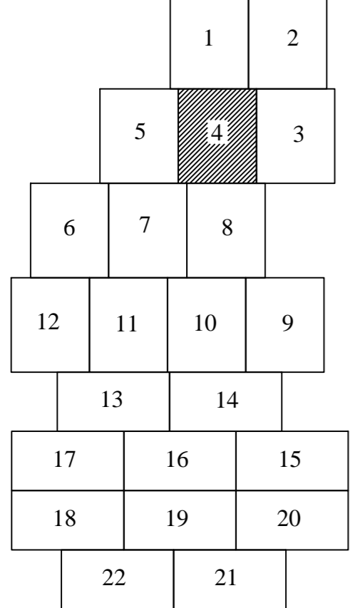
SCHEMA DE RACORDARE A PLANSELOR
