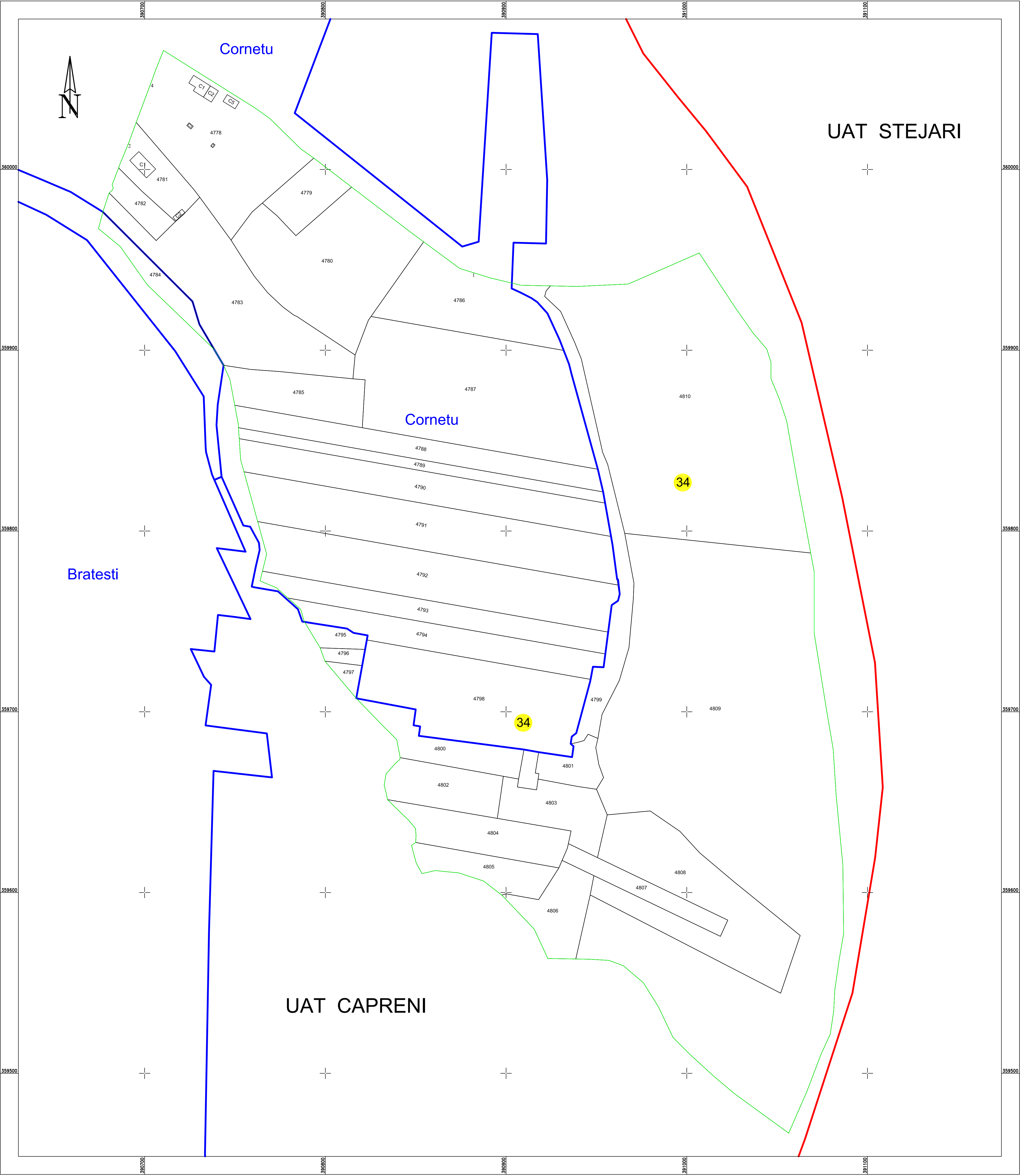
Schita cu disponerea sectoarelor cadastrale
