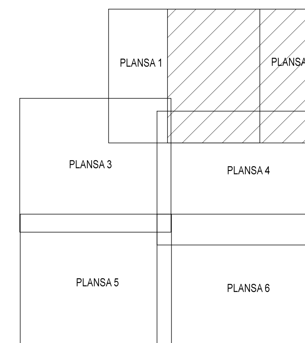
SCHITA DE RACORDARE A PLANSELOR
