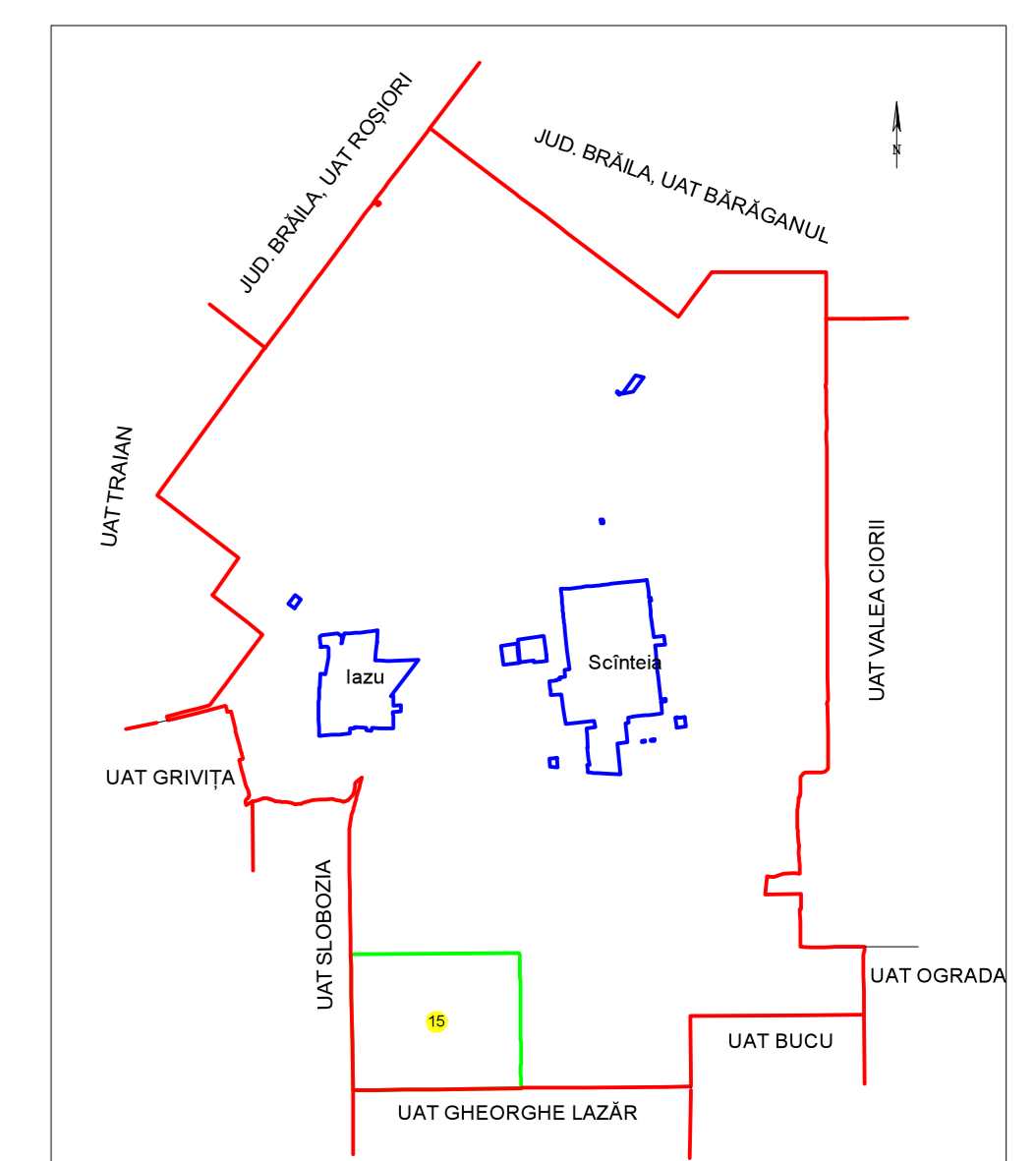
SCHITA DISPUNERII SECTORULUI CADASTRAL
