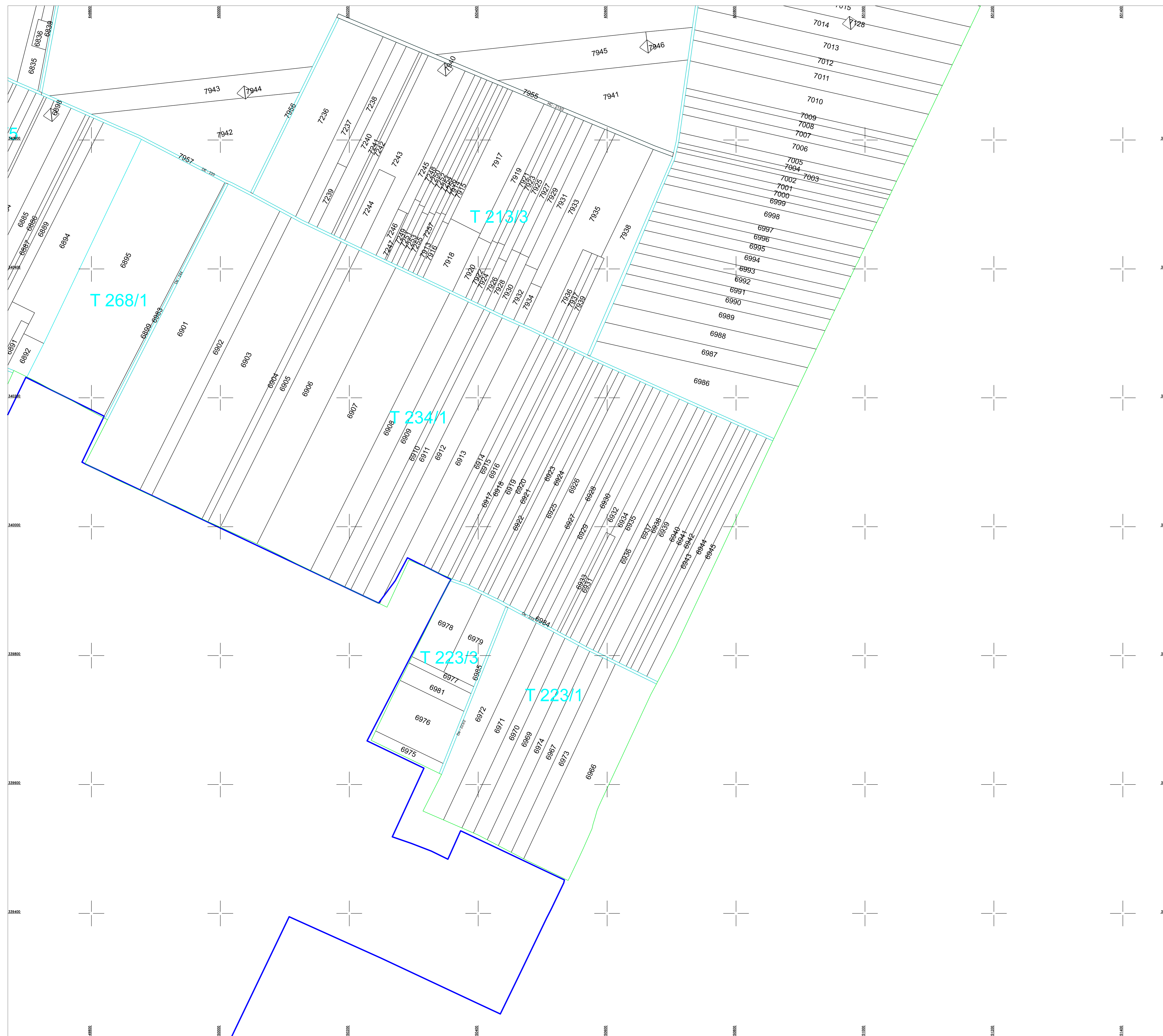
SCHITA DISPUNERII SECTORULUI CADASTRAL
