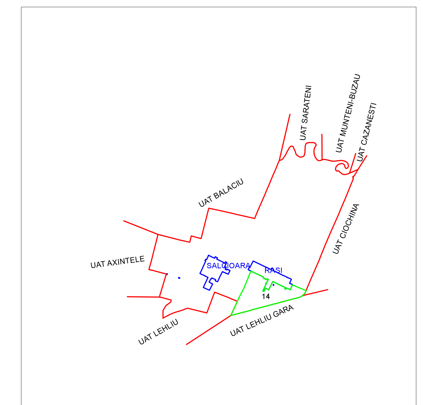
SCHITA DISPUNERII SECTORULUI CADASTRAL
