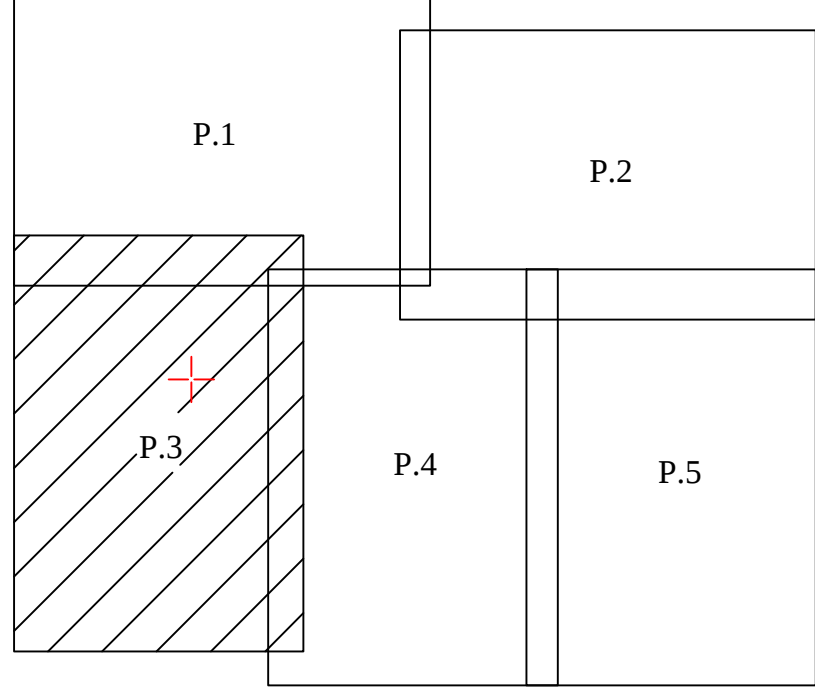
Schita de asamblare a planselor
