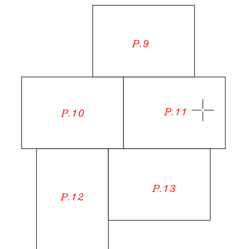
Schita de asamblare a planselor
