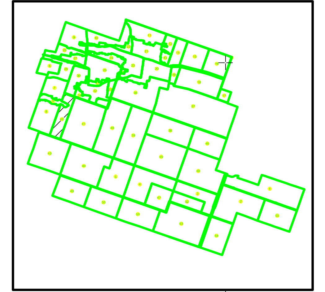
Schita cu dispunerea sectoarelor cadastrale
