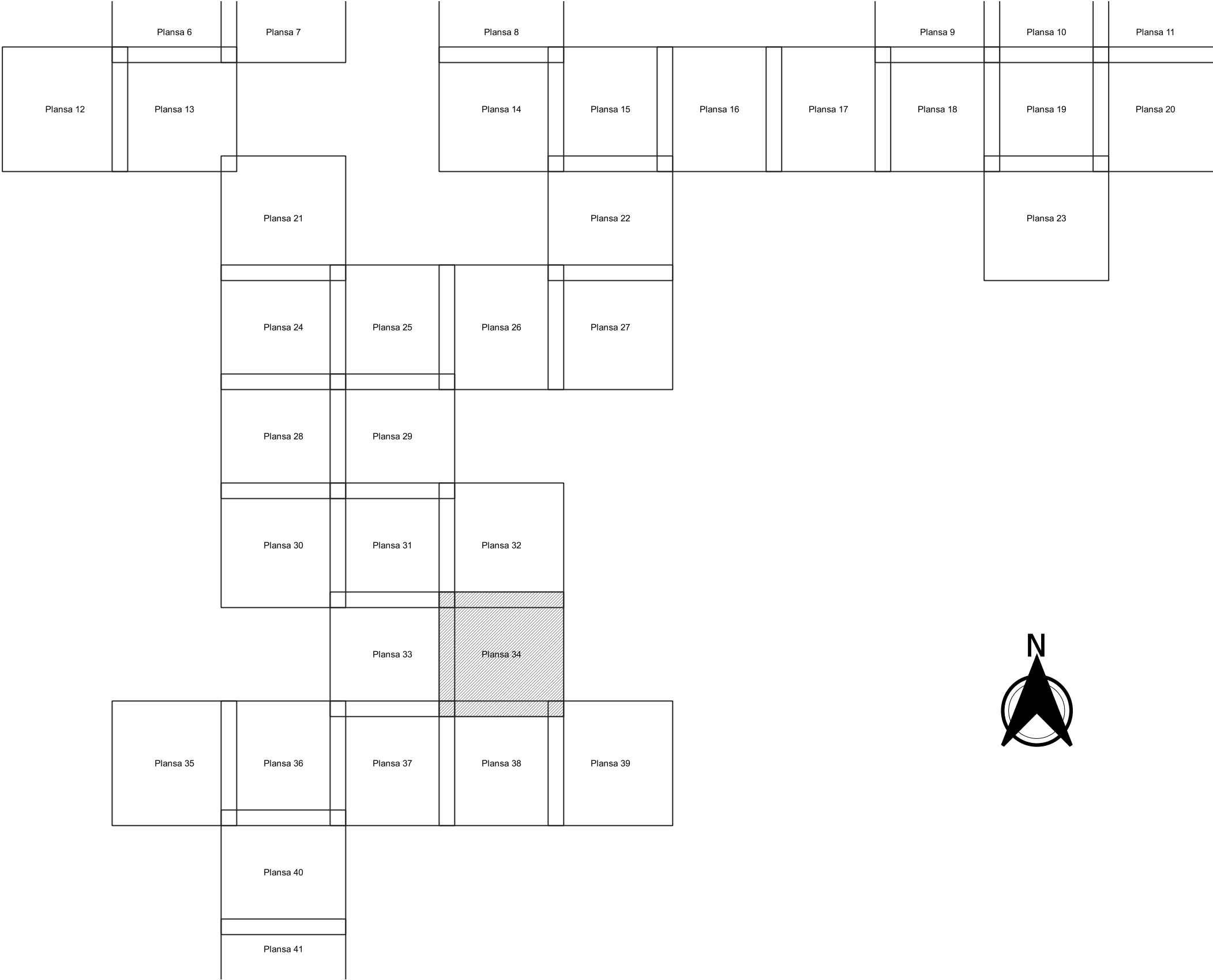
Schița de racordare a planșelor
